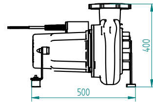
Trockenaufstellung
