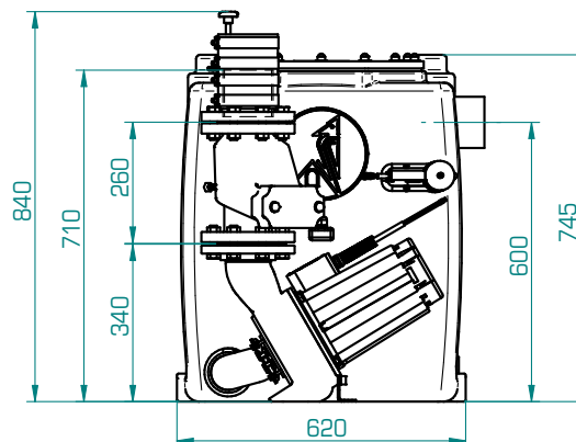
Baumaße HEBESTAR 400 STD
