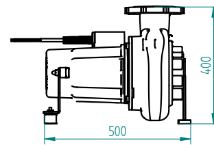
Trockenaufstellung
